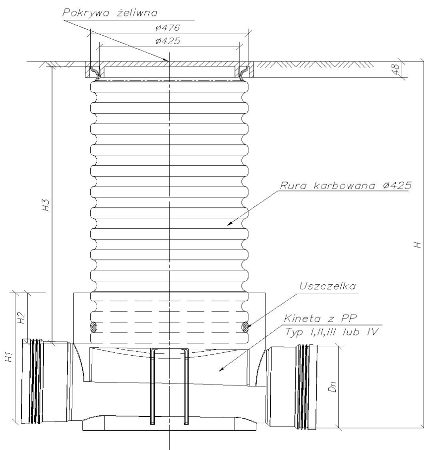
Studzienka inspekcyjna Ø425 z pokrywą żeliwną
